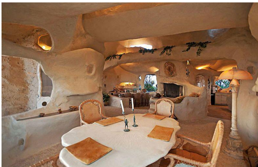
Maison troglodyte en béton de chaux et béton de chaux dans un chais viticole -©Jonathan BARBOT
